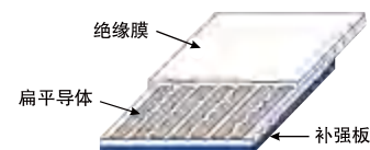
FFC产品的基本构造
